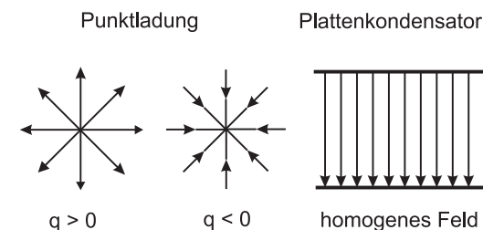
Abbildung 1.3: Beispiele für von Ladungen erzeugte Felder.
