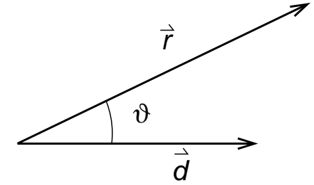
Abbildung 1.7: Winkel zwischen Beobachtungspunkt \vec{r} und Dipolmoment \vec{d} .
