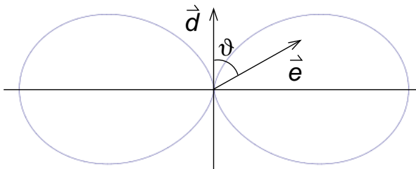
Abbildung 12.1: Charakteristische Winkelabhängigkeit der Dipolstrahlung.
